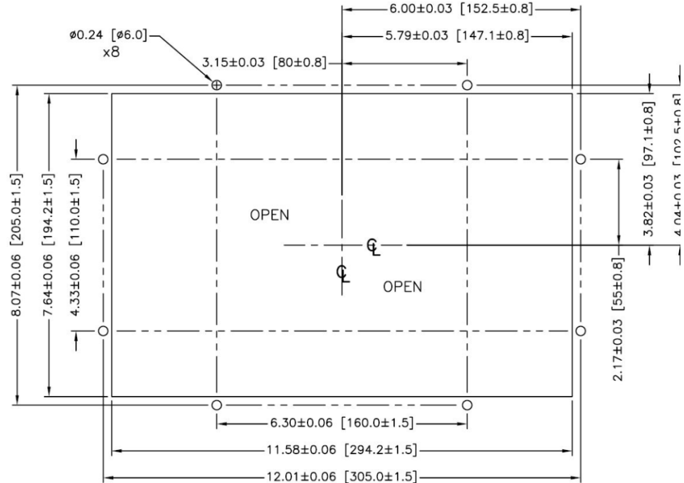
Abbildung 2-4: Plattenausschnittabmessungen
