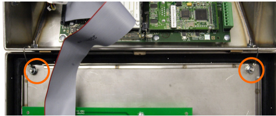
Figure 2-8: Emplacements de fixation des bandes de mise à la terre
