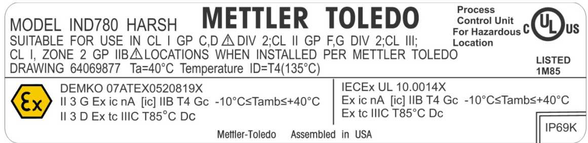
Figure 1-1: Étiquette de données, enceinte pour environnement rude, ATEX/IECEx
