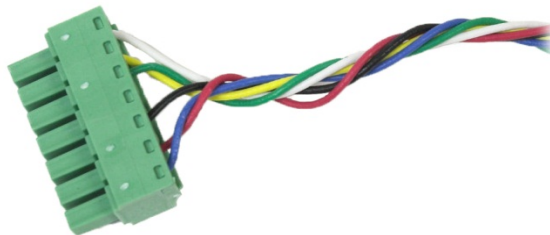
Abbildung 2-18: Zusammengedrehte Optionsplatinendrähte
