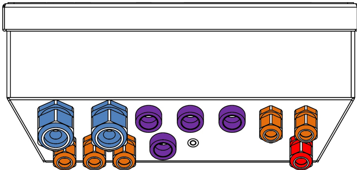
Figura 2-19: Asignaciones de las aberturas para cables en cajas para ambiente adverso
