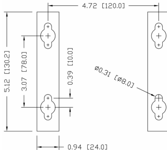
Figure 2-12: Emplacement des trous de montage
