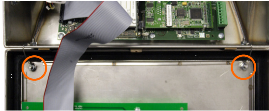
Abbildung 2-8: Positionen der Befestigung des Erdungsbands
