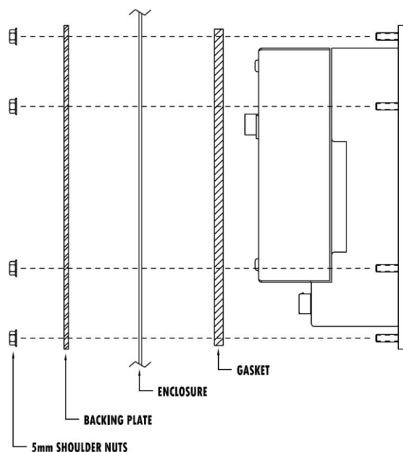
Figura 2-6: Montaggio a pannello, vista laterale
