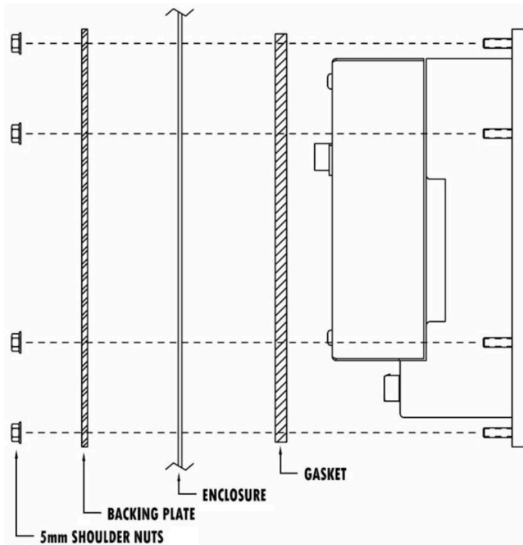
Figura 2-6: Montaje en panel, vista lateral
