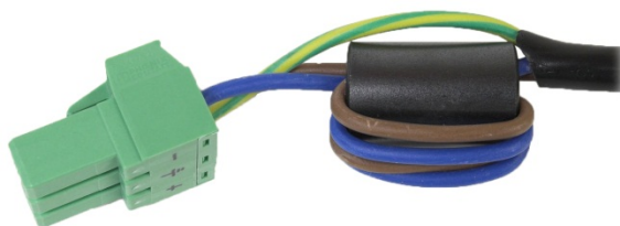
Figura 2-16: Nucleo in ferrite sul cavo di alimentazione per montaggio a pannello
