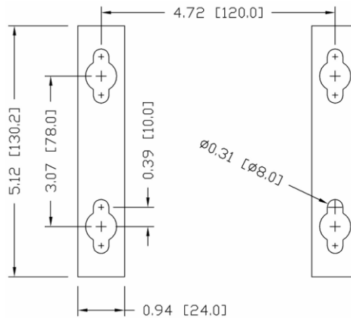
Figura 2-12: Forometria per il montaggio
