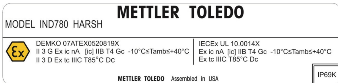
Figura 1-1: Etichetta di omologazione, armadietto per ambienti difficili, ATEX/IECEx
