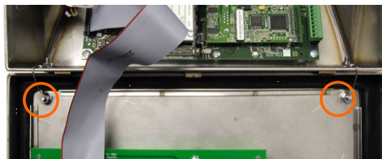
Figura 2-8: Posizioni di attacco della piastrina di massa
