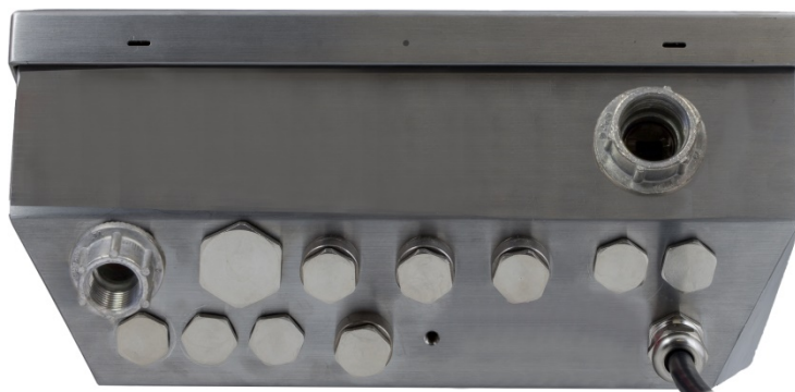
Figura 2-1: Installazione snodo per canalina, armadietto per ambienti difficili
