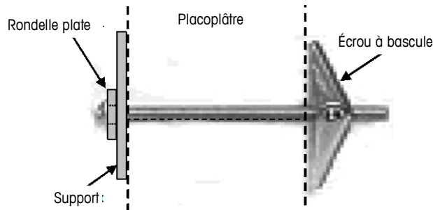
Figure 2-15: Installation sur panneau de revêtement ou placoplâtre
