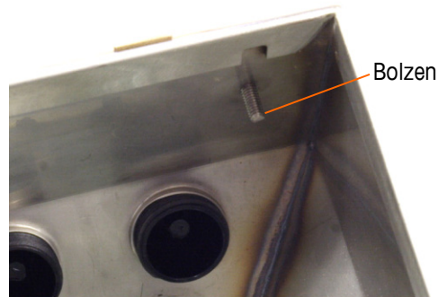
Abbildung 2-9: Bolzen zum Anbringen der umgekehrten Frontplatte
