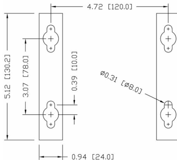
Abbildung 2-12: Montagelochmuster
