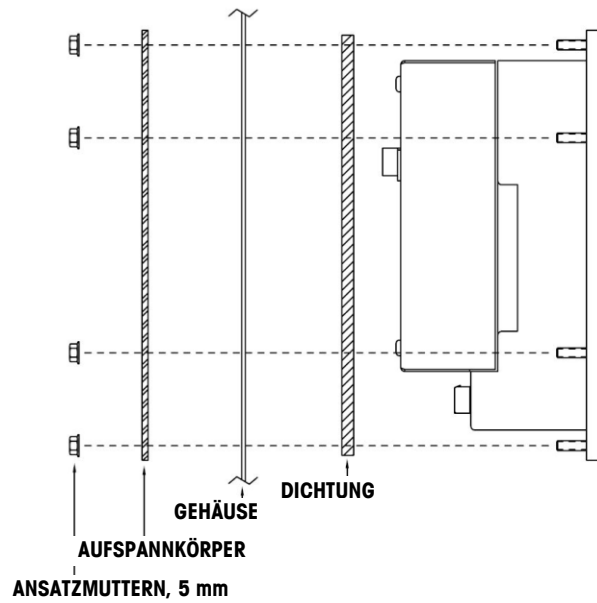
Abbildung 2-6: Schalttafelmontage, Seitenansicht
