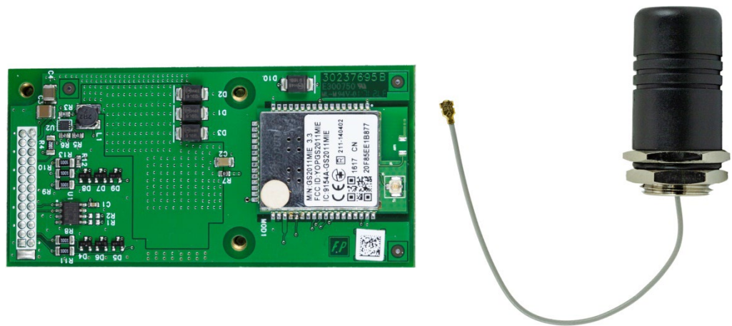
Figura 2-16: Placa de Opção de WiFi e Antena da IND256x
