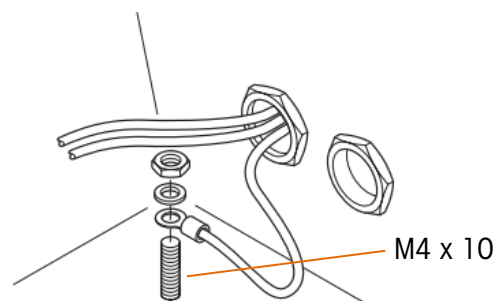
Figure 2-9 : Connexion du câble blindé à la borne
